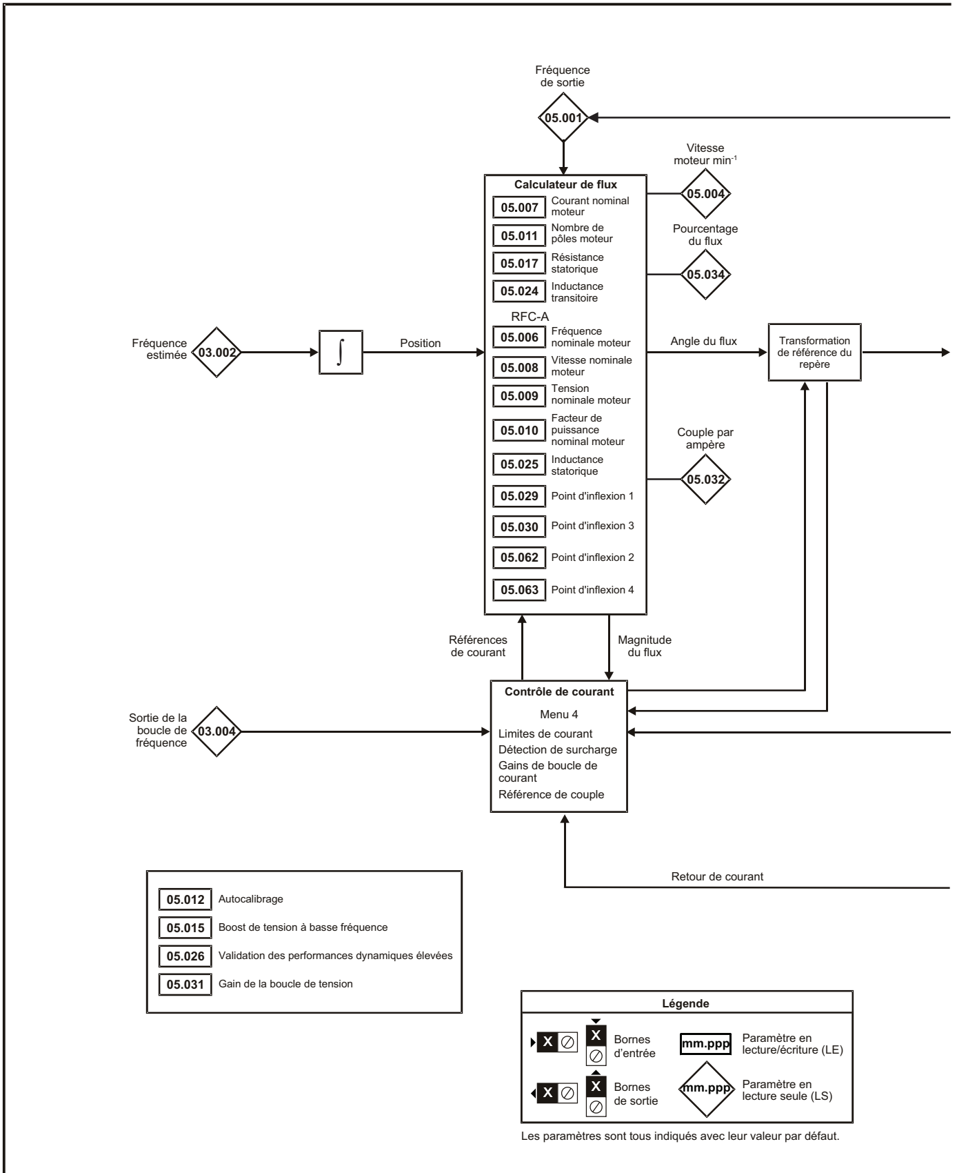
Figure 11-13 Schéma logique du menu 8
