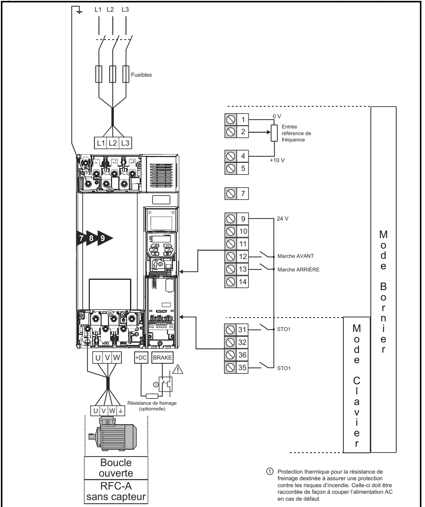
Figure 7-4 Connexions minimales pour la mise en marche du moteur dans tous les modes de fonctionnement (taille 7 et supérieures)
