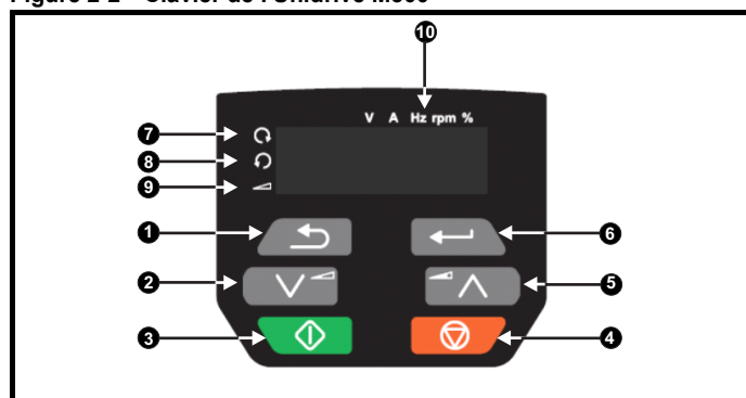
Figure 2-2 Clavier de l'Unidrive M300
