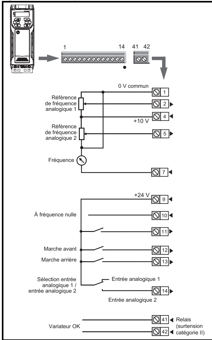
Figure 4-3 Fonctions par défaut des bornes
