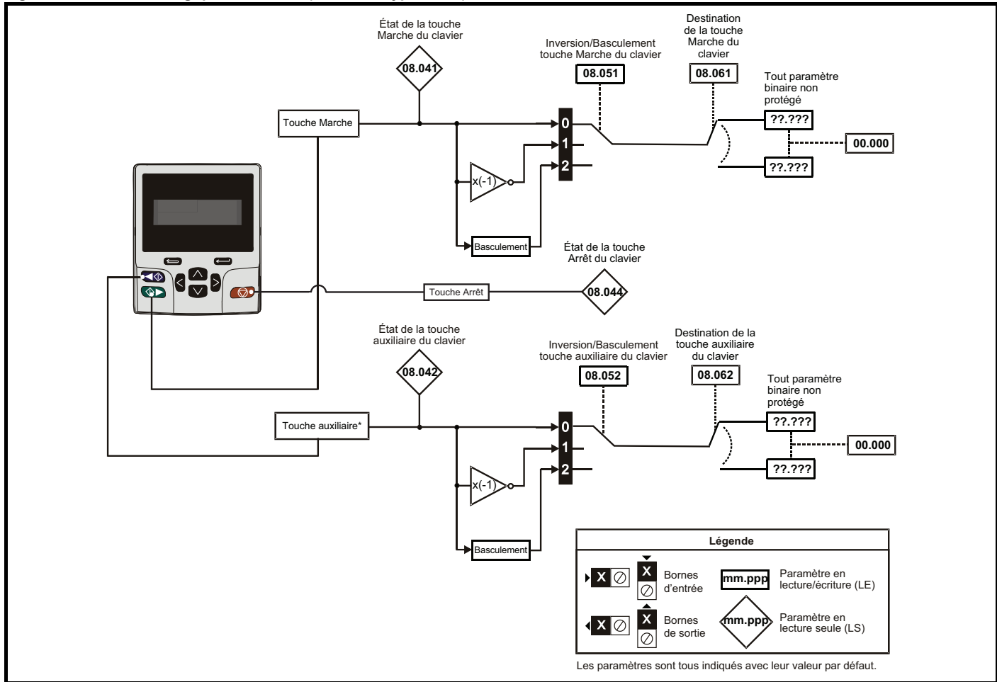
Figure 11-17 Schéma logique du menu 8 (Remote Keypad RTC)
