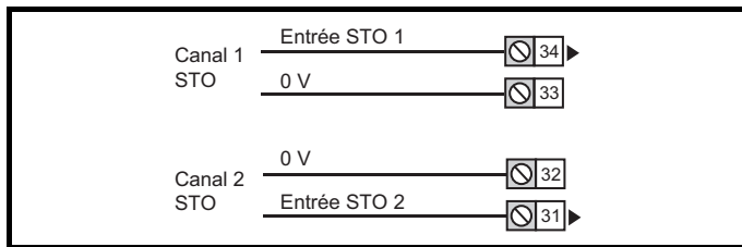
Figure 4-5 Entrées Absence sûre du couple (Tailles 5 à 9)
