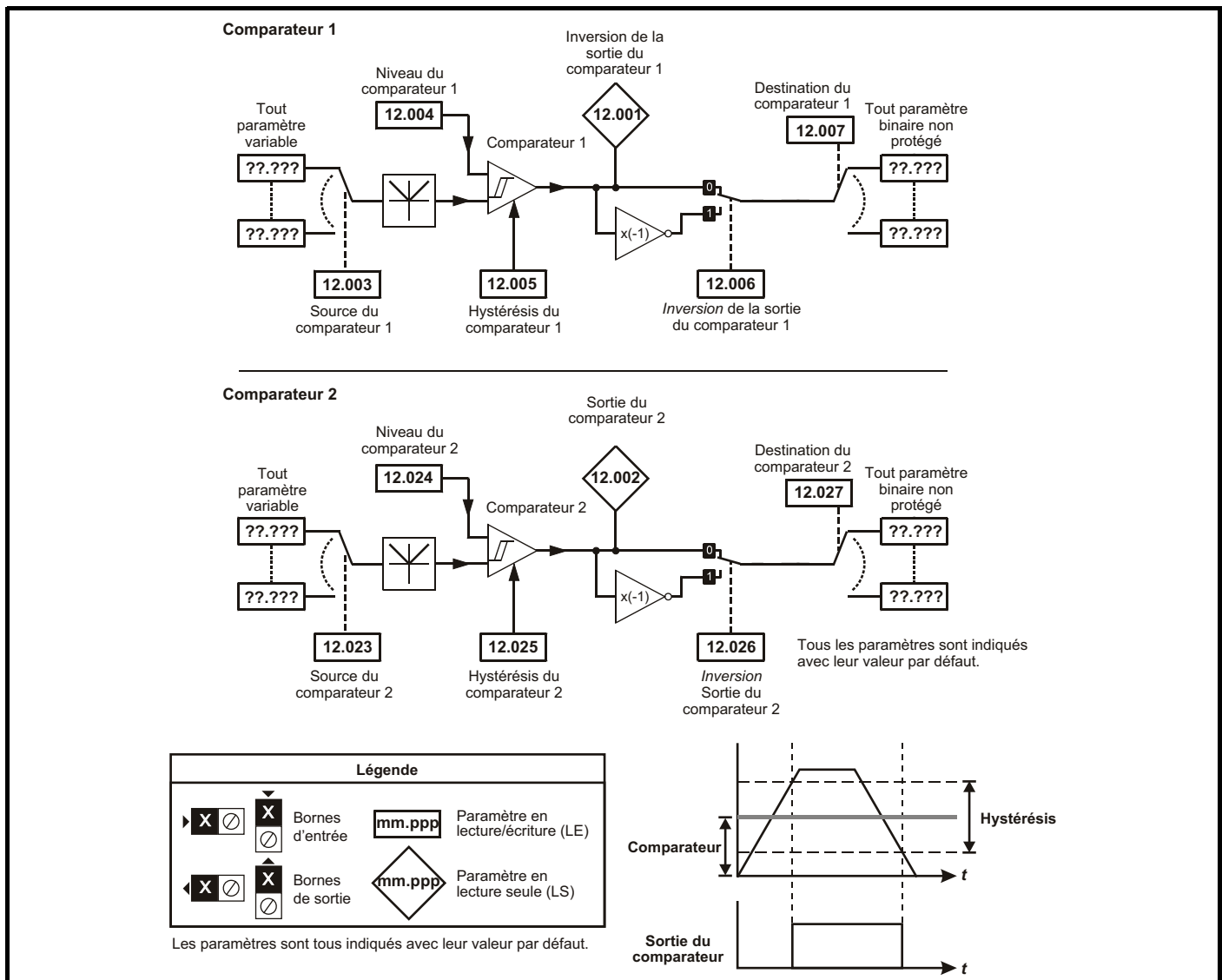
Figure 11-21 Schéma logique du menu 12
