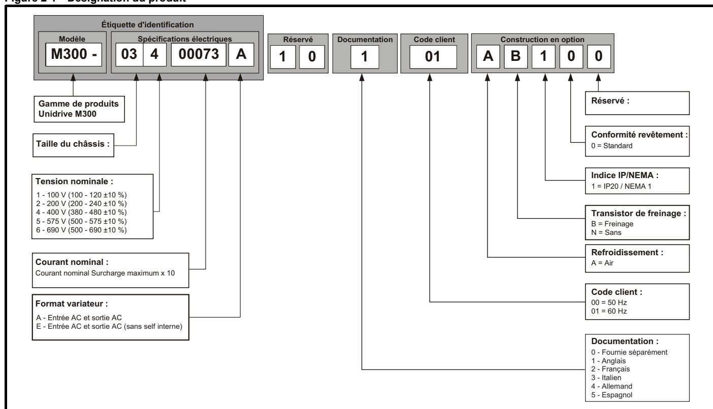
Figure 2-1 Désignation du produit
