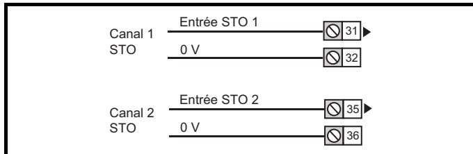
Figure 4-5 Entrées Absence sûre du couple (Tailles 5 à 9)
