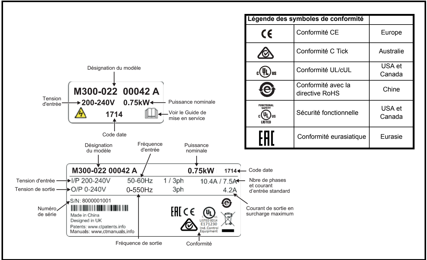
Figure 2-3 Étiquettes standard du variateur taille 2
