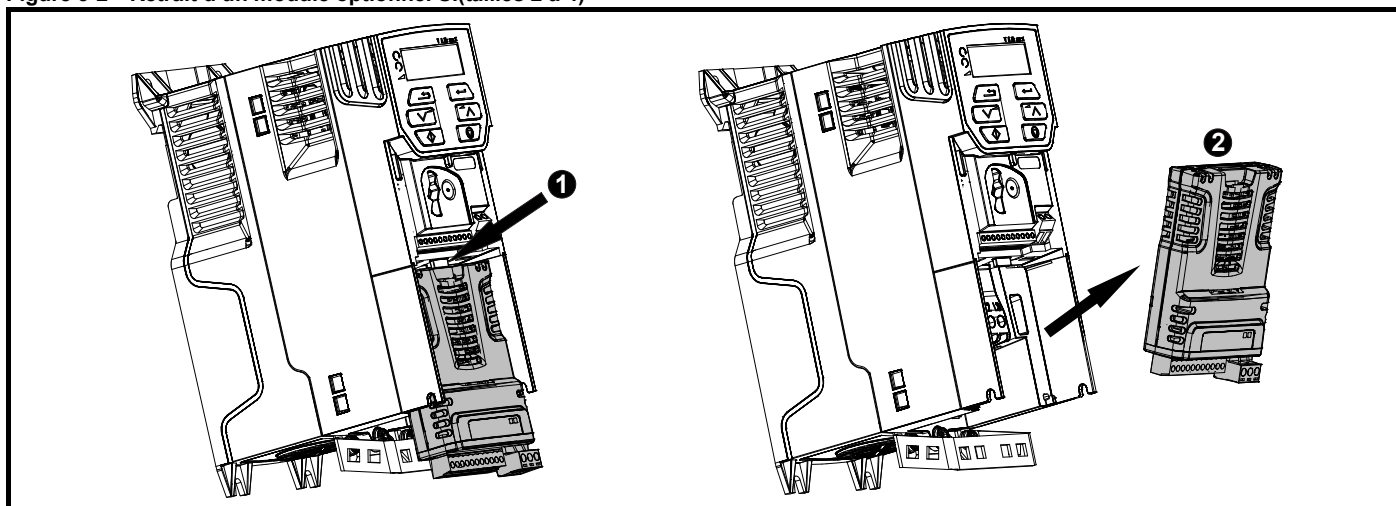
Figure 3-2 Retrait d'un module optionnel SI(tailles 2 à 4)
