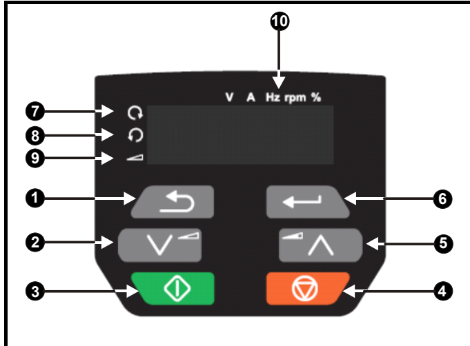
Figure 5-1 Caractéristiques de l'afficheur
