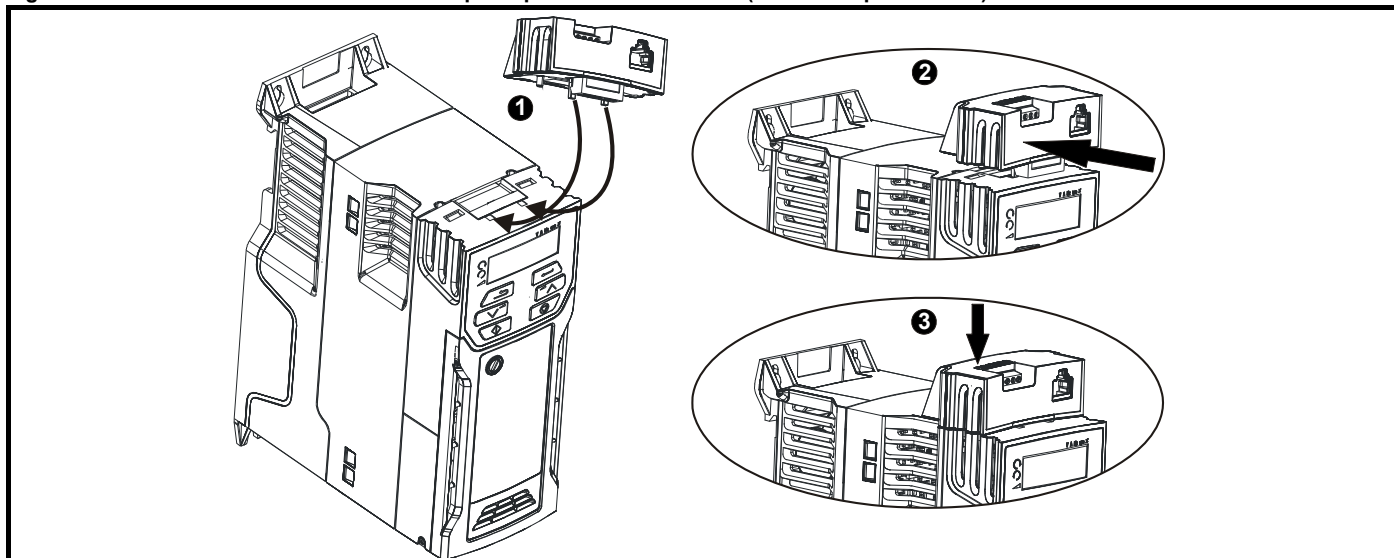
Figure 3-5 Installation de l'AI-485 / AI-Backup Adaptor dans le variateur (AI-485 Adaptor illustré)
