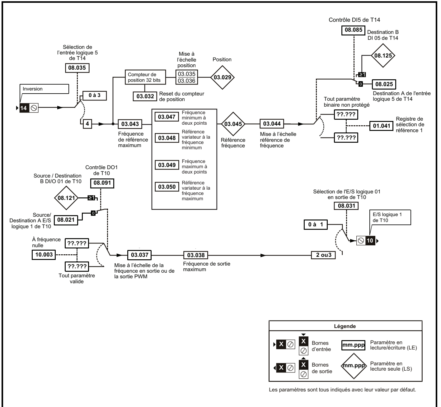
Figure 11-5 Schéma logique du menu 3
